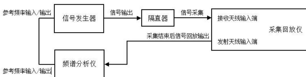
图 3 采集带宽测试图
