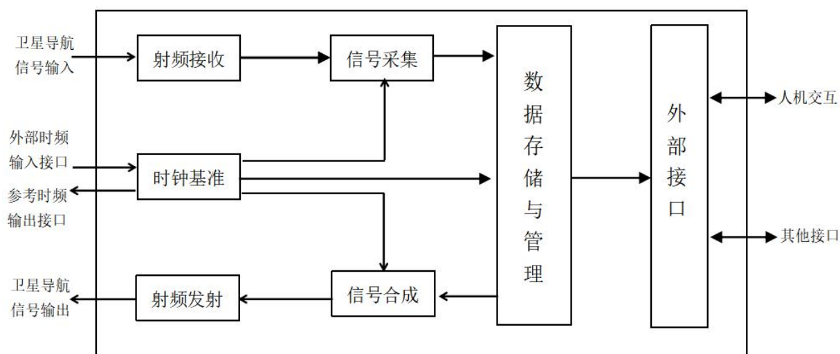
图 1 采集回放仪结构示意图
