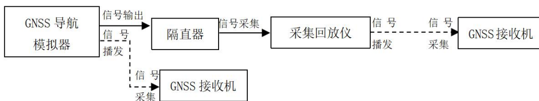
图 7 伪距准确度测试图
