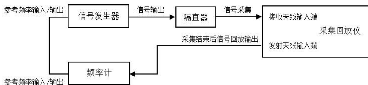
图 4 回放信号频率偏差测试图
